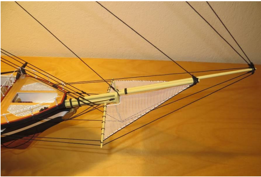
Montering af bovspyd.
