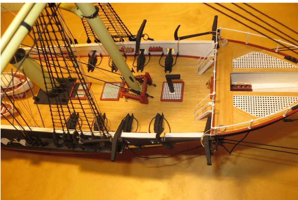
Montering af ankre.
